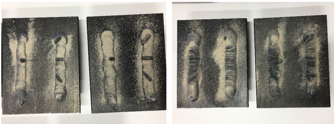
Bild 4: Klebestränge mit Quarzsandauflage, nach (a) Aufsitzen und (b) Trippeln
