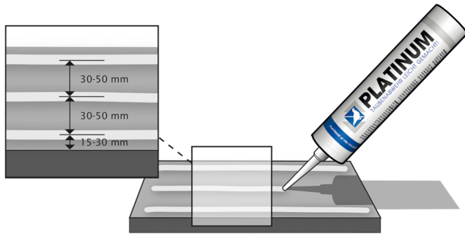
Vorschlag zur Aufbringung auf kleineren ebenen Flächen.
