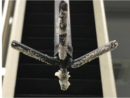
Bild 5: Taubenfüße nach Test mit Quarzsandauflage, nach (a) Aufsitzen bzw. (b) Trippeln
