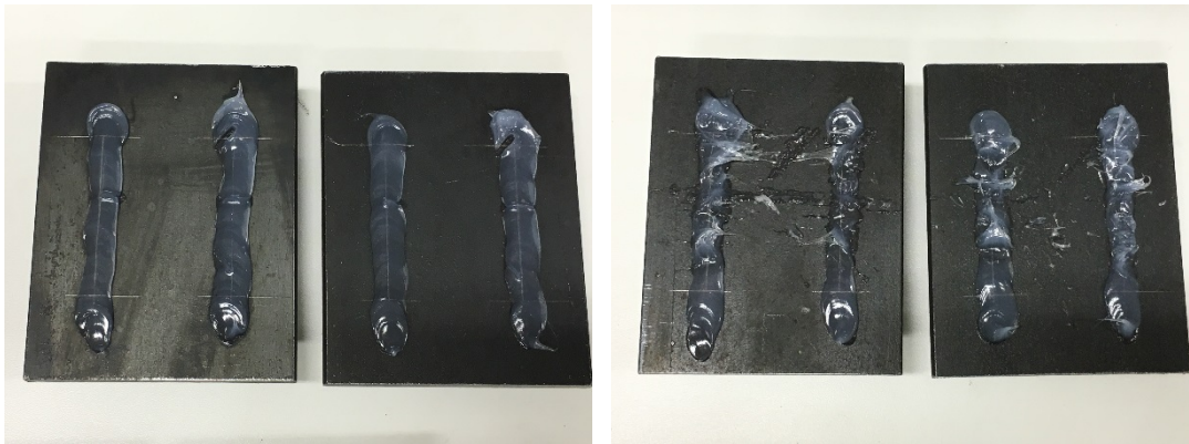
Bild 2: Klebestränge ohne Quarzsandauflage, nach (a) Aufsitzen und (b) Trippeln
